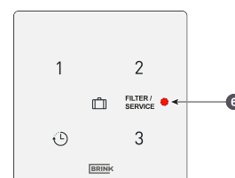
6 = LED (blinker 0,5 sek. tændt - 60 sek. slukket)
